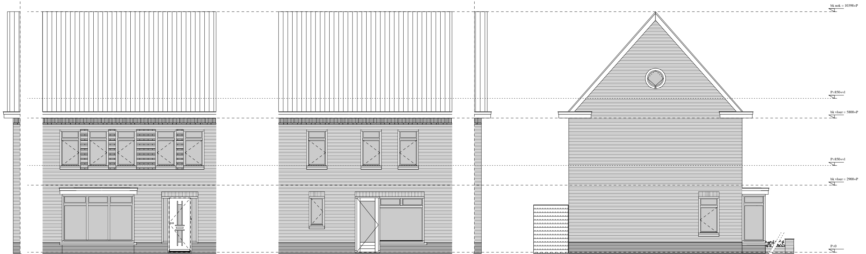
zijgevel
